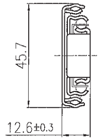
A視圖 (2:1)
